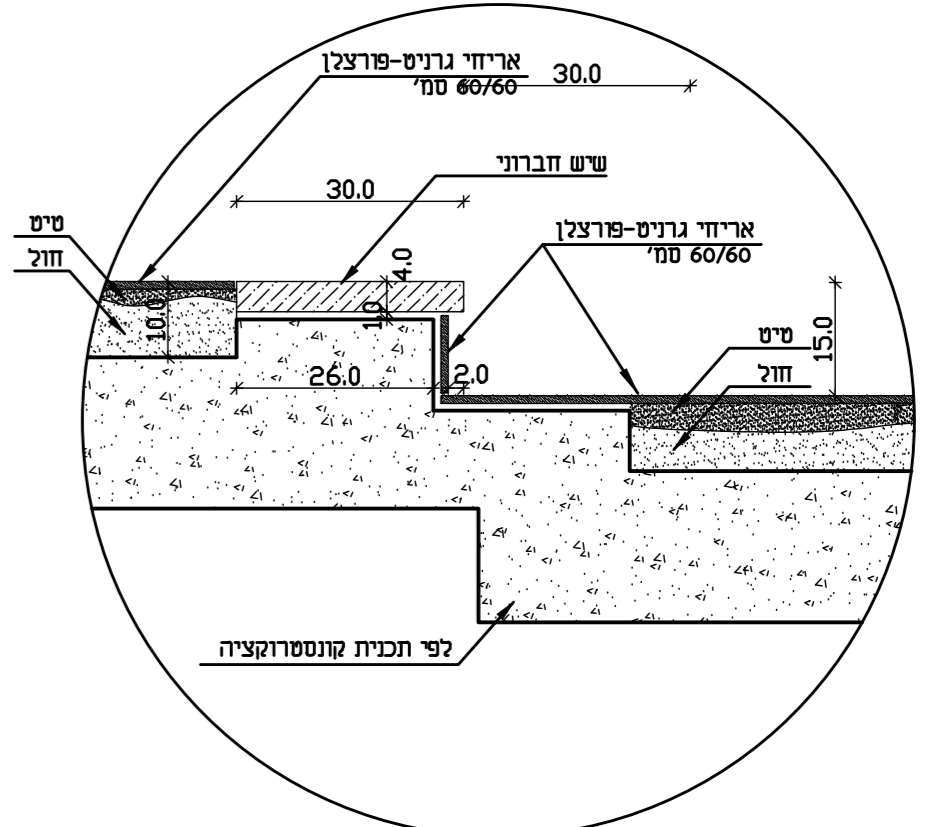
חיתך 2-2
