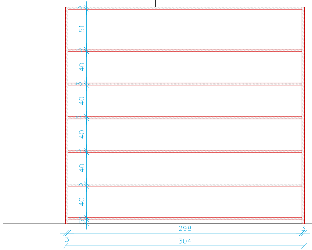
חזית א
