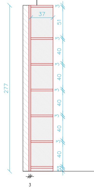
חתך א-א
