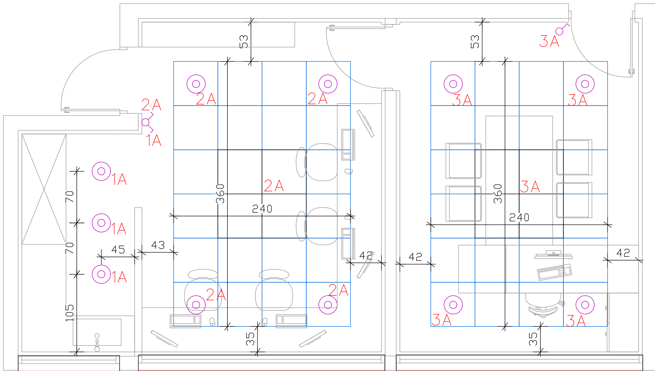
תוכנית תקרה פריקה וגבס קנ"מ 1:50
