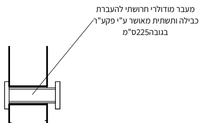
חתך
