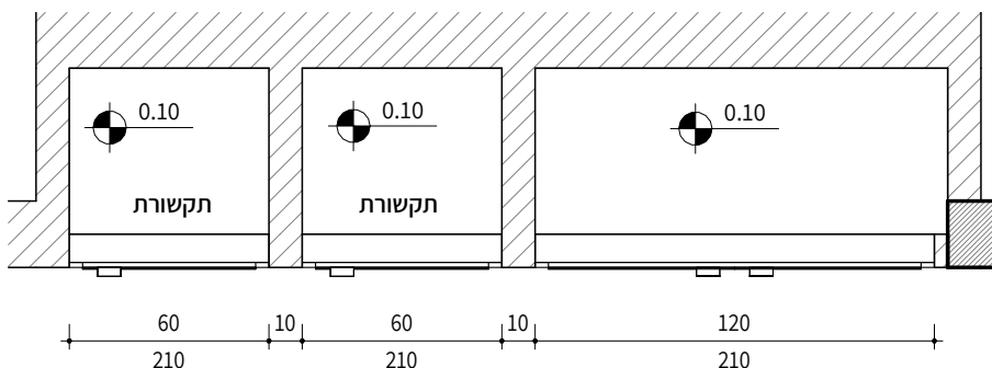
תכנית
