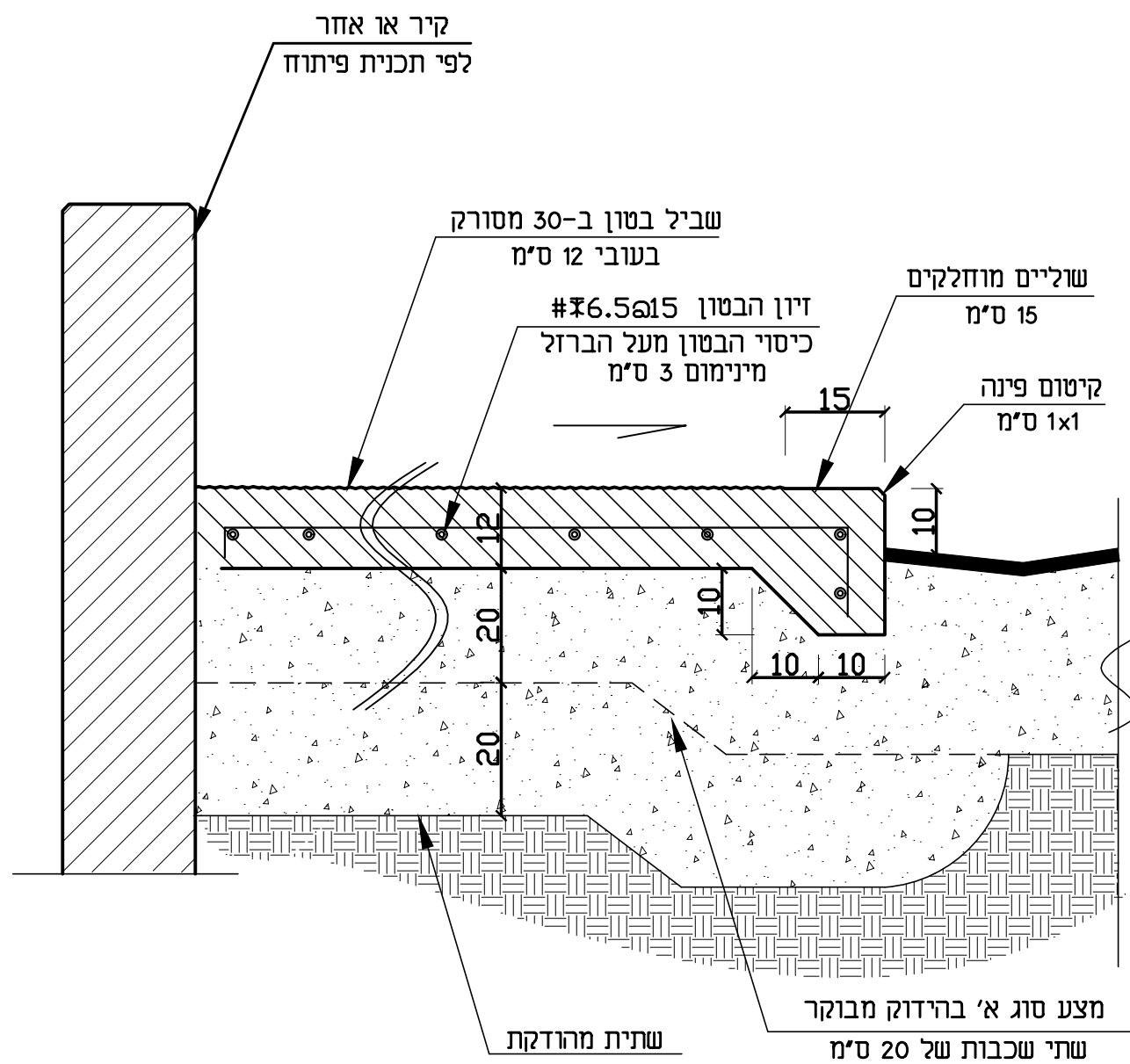
חתך אופייני קני"מ 1:10
