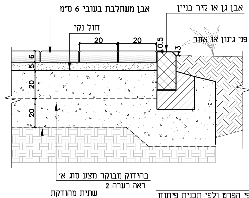
חתך עקרוני קנ"מ 1:10
