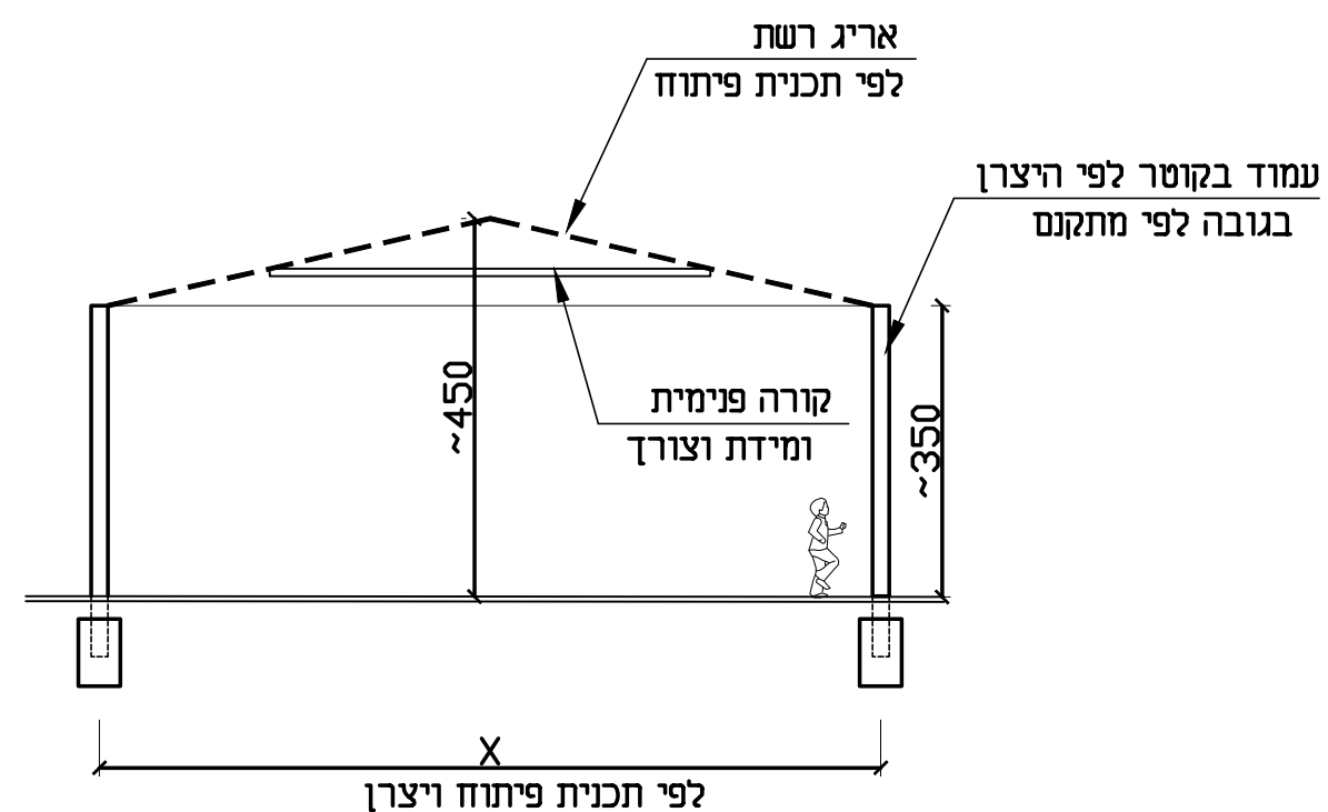
חתך עקרוני קני"מ 1:100
