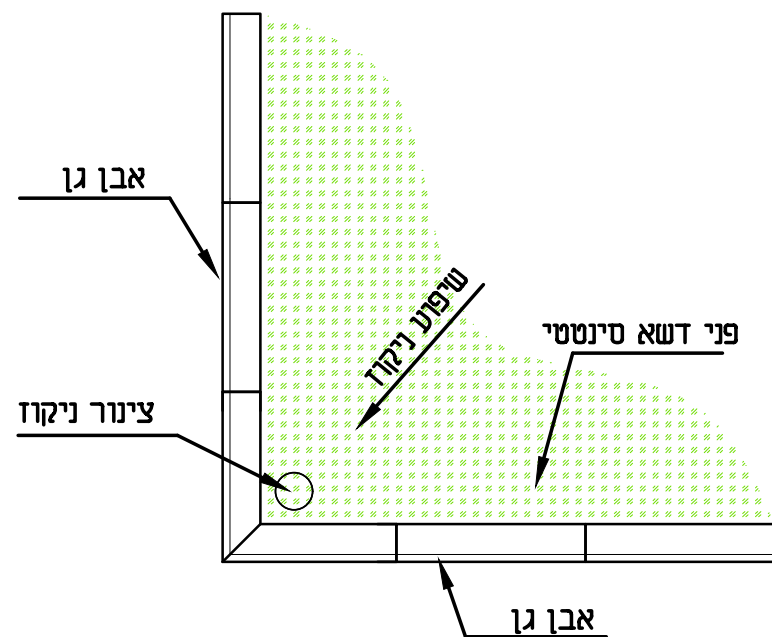
פרט ניקוז - פתח באבן גן תכנית קנ"מ 1:20
